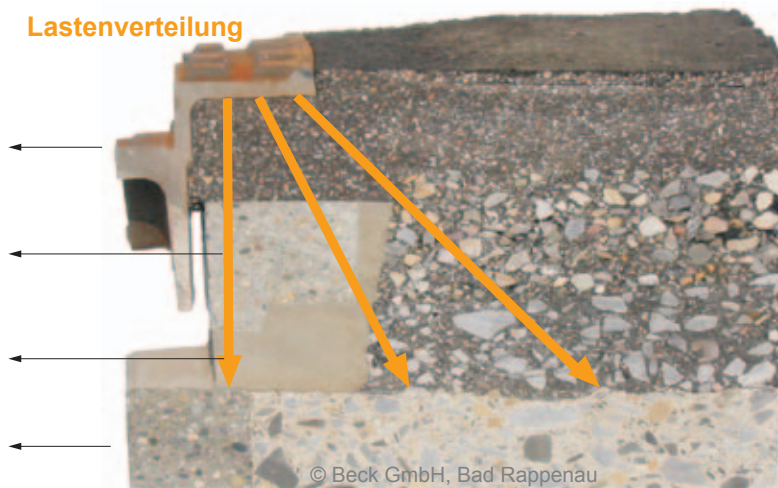
Schachtabdeckung, LW 605, Klasse D 400, System Bituplan®, Rahmen aus Gusseisen, BEGU®-Deckel nach DIN 19584 mit Lüftungsöffnungen
